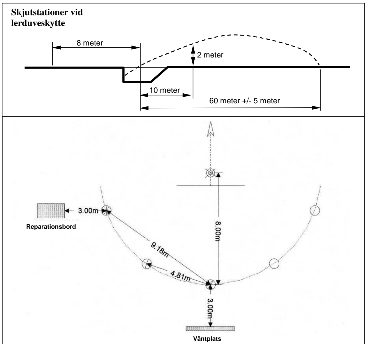
Figur 1. Skjutstationens utformning.
